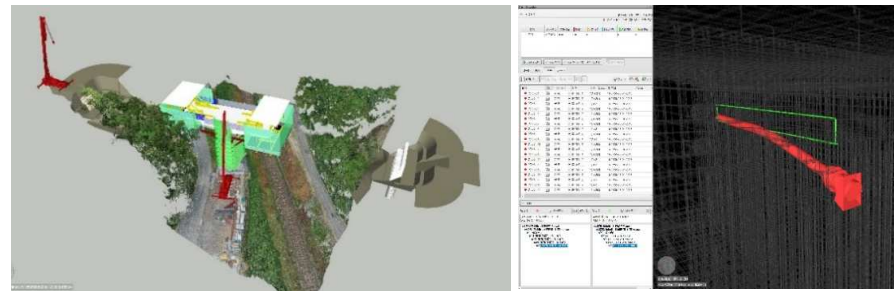
実工程に合した4D施工シミュレーション
