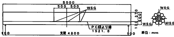
図-6 ワイヤーストレインゲージ位置
