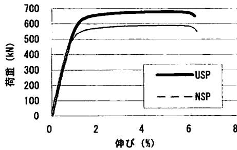
図-1 荷重～伸び関係
