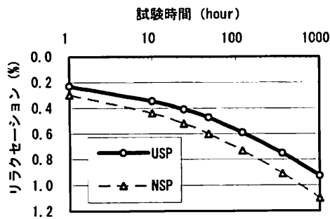
図-2 リラクセーション試験結果
