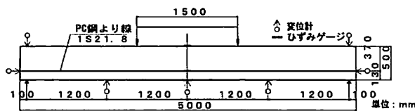
図-7 載荷位置および計測位置
