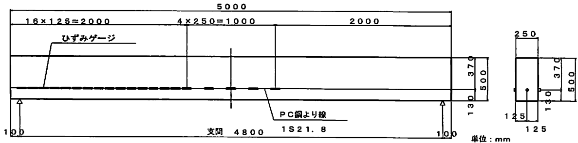
図-5 コンクリートゲージ位置
