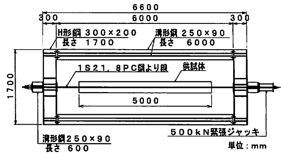
図-4 供試体製作設備
